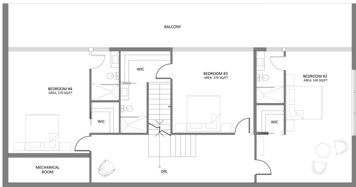
Demi sous-sol / Semi-basement
